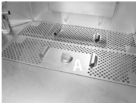
εικόνα 24 Σχάρες δεξαμενής
