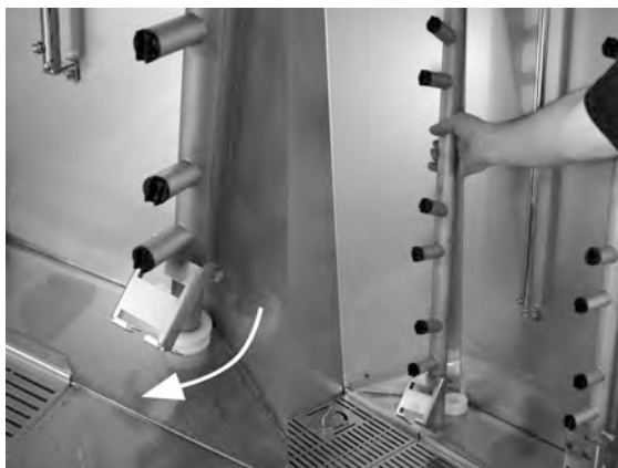
Photo 22 Enlevez les buses de lavage
