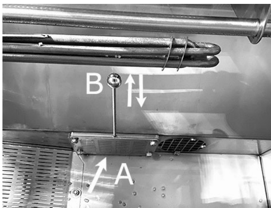
obraz 39 Sito do pompy do mycia naczyń
