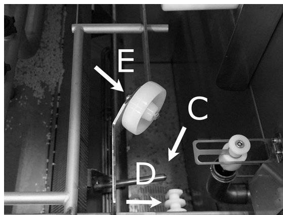
obraz 38 Dolne sito, czujnik poziomy oraz wałki
