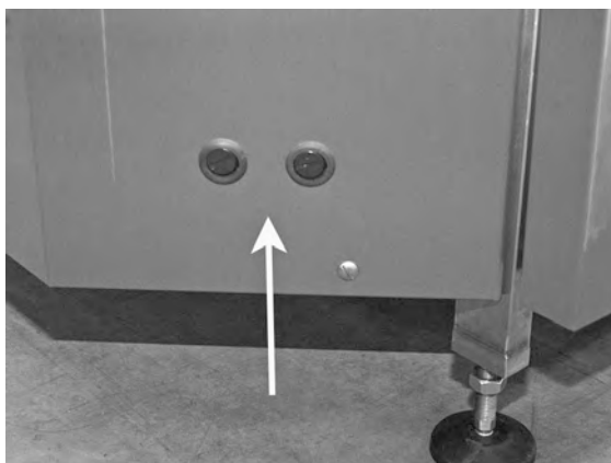
Imagen 18 Acceso a los protectores contra sobrecalentamiento
