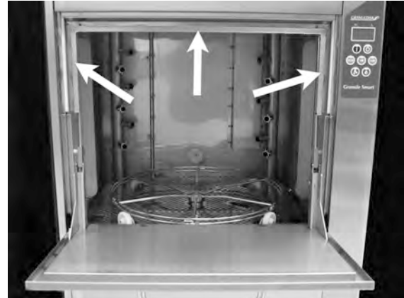
Fig. 40 Letisztítandó ajtókeret
