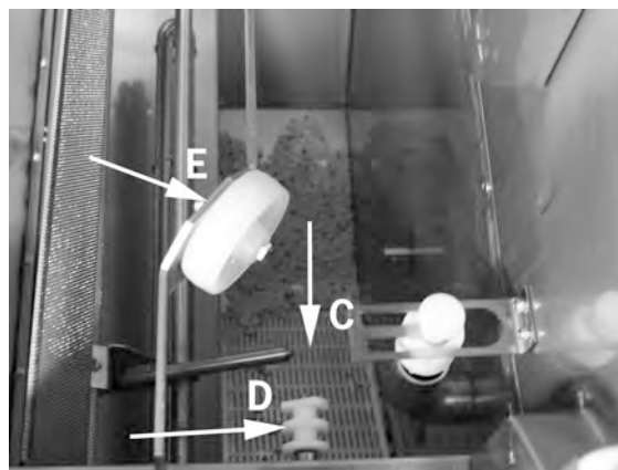
Fig. 36 Az alsó szita, a szintérezékelő és a görgők
