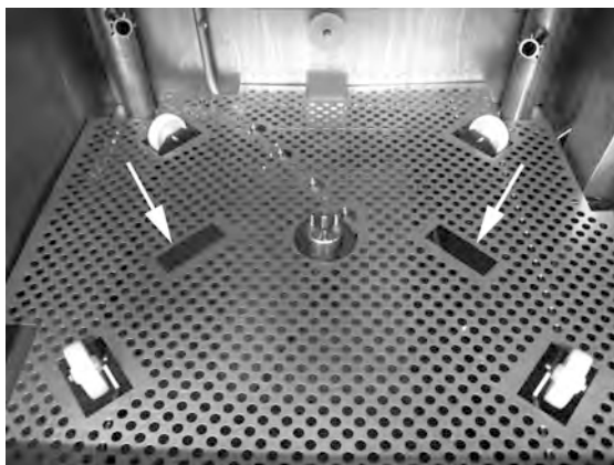
Fig. 34 Tartályrács
