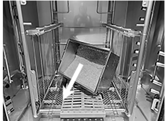
Kuva 3 Rakeiden lisääminen
