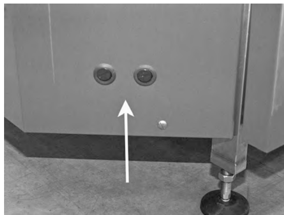
Bilde 18 Overopphetingsvern
