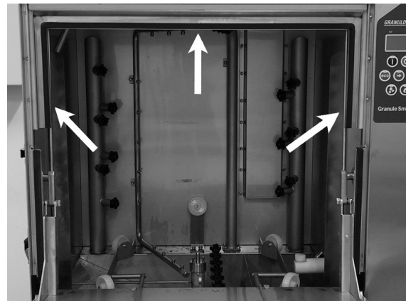
Fig. 43 Door frame to clean
