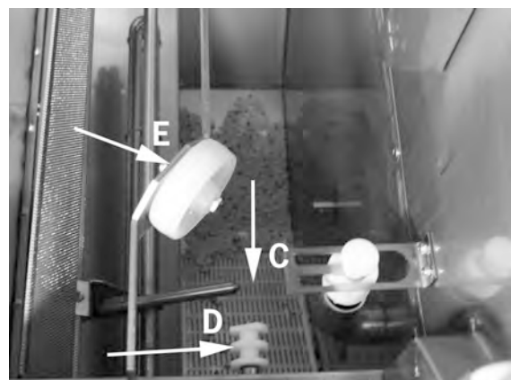
Billede 36 Bundsigte, niveausensor og ruller
