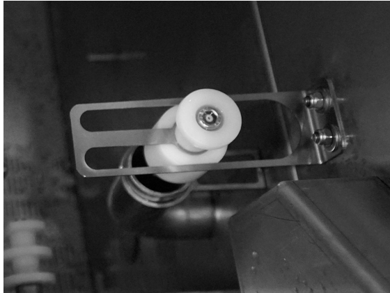
Abbildung 37 Überlaufarmatur
