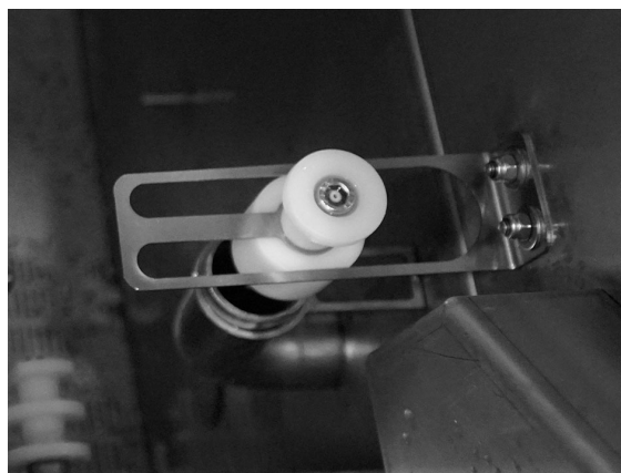
Afbeelding 40 Overloopkraan
