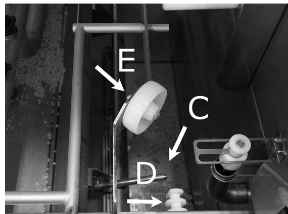
Afbeelding 38 Bodemzeef, niveausensor en roller
