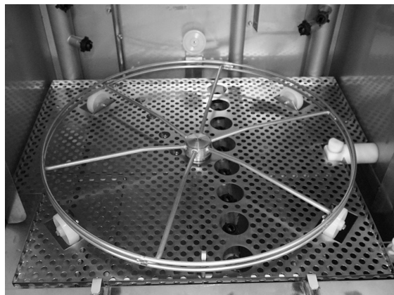
Afbeelding 35 Korfwiel
